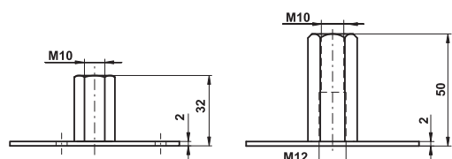
ZB N V4A
