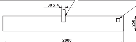
ZD 01 - s navařenou zemní páskou délky 6m, ZD 01a - se svorkou (pro 30x4 a ø 8-10)
